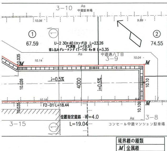
路計画平面図
