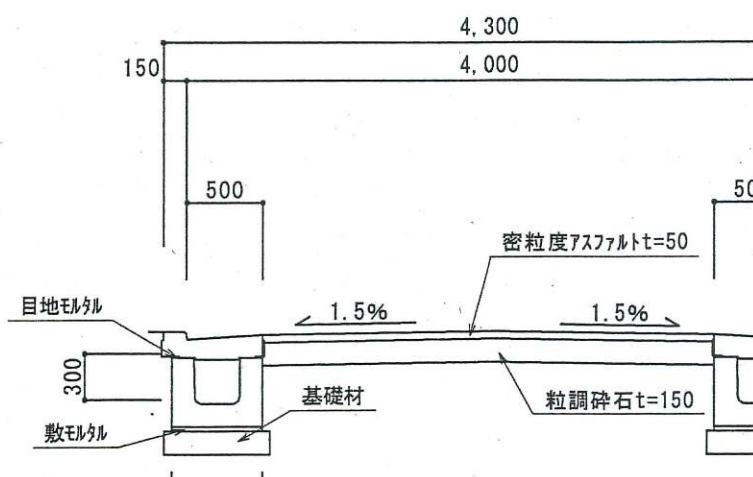
標準横断面図(b-b') S:1
