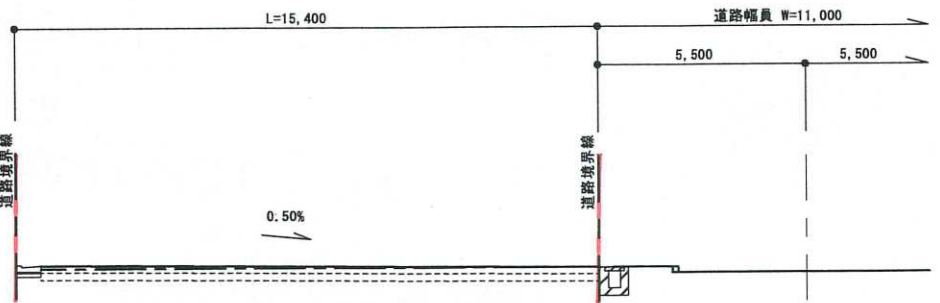
道路縦断面図 S=1/200
