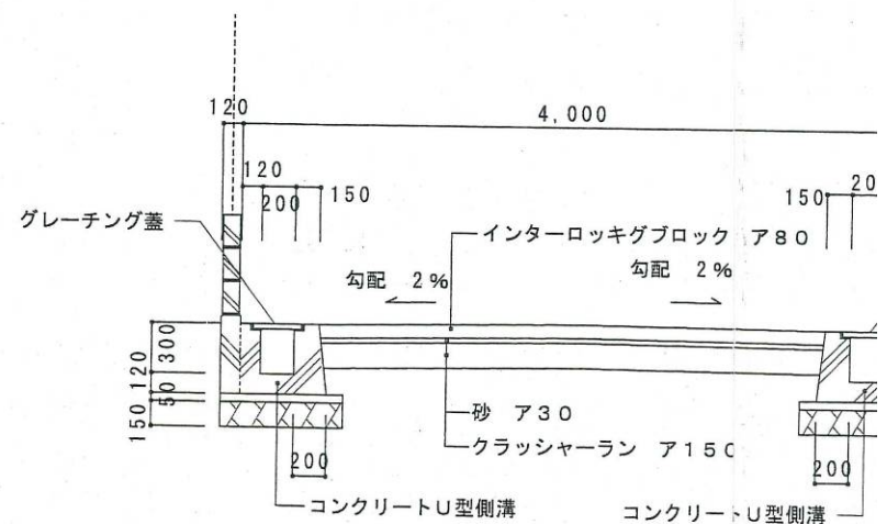
標準横断面図 1/50
