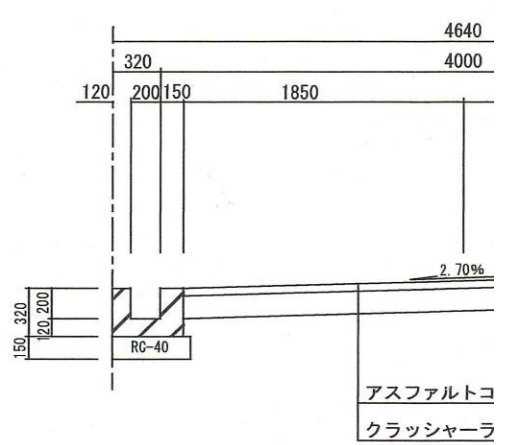
標準横断面図 (S=1:50)
