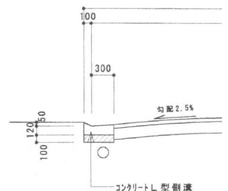
標準横断面図 (S=1:50)
