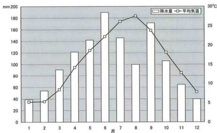
図 2-3 月別の平均気温と降水量の推移
